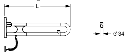
Wandanschluss mit 2 E-Taster Wall mounting with 2 E-Buttons
