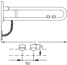
Wandanschluss mit 2 E-Taster Wall mounting with 2 E-Buttons
