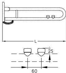
Anschluss verdeckt mit Montageplatte mit 2 E-Taster Connection to mounting plate with 2 E-Buttons
