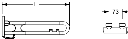
Anschluss verdeckt mit Montageplatte mit 2 E-Taster Connection to mounting plate with 2 E-Buttons
