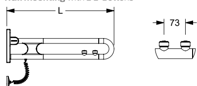
Wandanschluss mit 2 E-Taster Wall mounting with 2 E-Buttons
