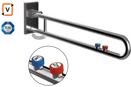
Anschluss verdeckt mit Montageplatte mit 1 E-Taster Connection to mounting plate with 1 E-Button
