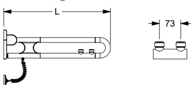
Wandanschluss mit 2 E-Taster Wall mounting with 2 E-Buttons
