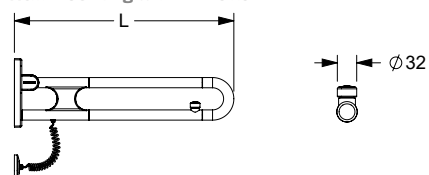
Wandanschluss mit 2 E-Taster Wall mounting with 2 E-Buttons
