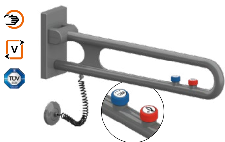
Wandanschluss mit 1 E-Taster Wall mounting with 1 E-Button
